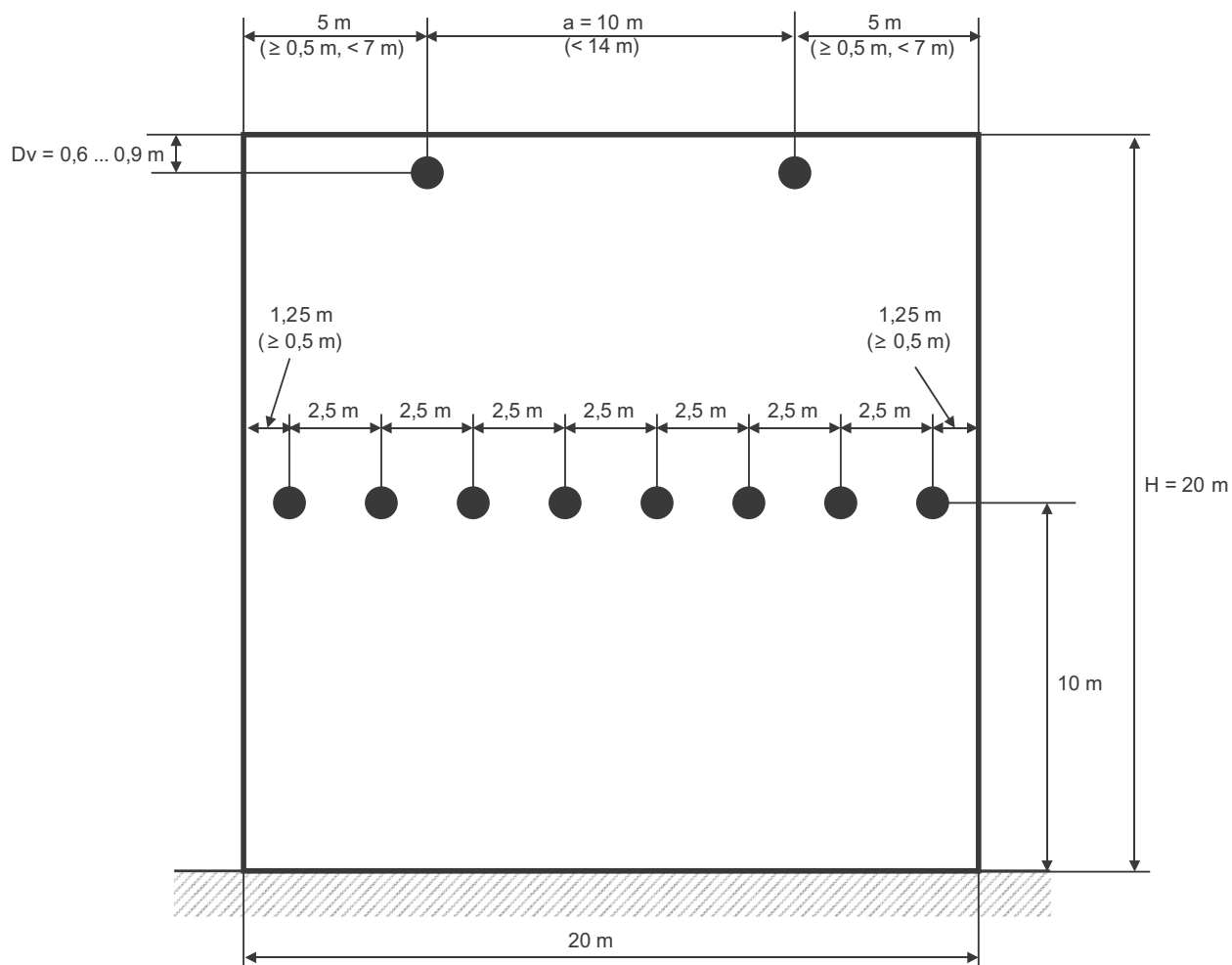
Fig. 3.20 Exemplu de amplasare a unor detectoare liniare de fum într-o incintă cu înălțimea de 20 m (vedere perpendiculară pe direcția fasciculelor de detectare)
